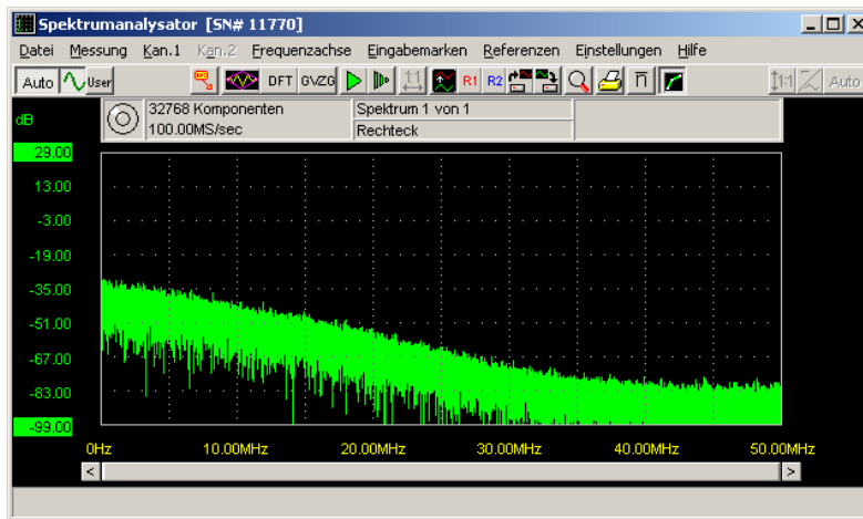
Abbildung: Typisches 1/f-Rauschen nach der Verstärkung
